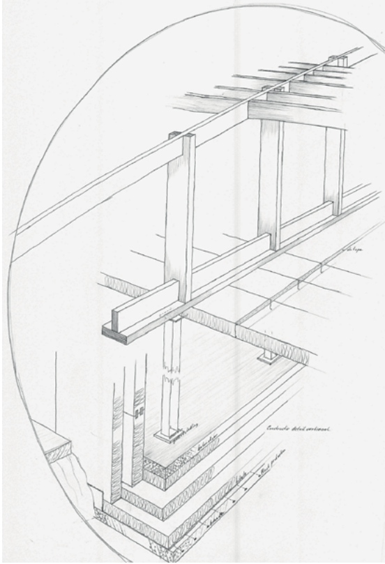
Abbildung 5 Detail der vertikalen Dachkonstruktion
