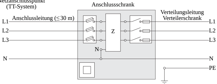
Bild 6.5 Anschlussbeispiel von Baustromverteiler im TT-System (Quelle: VDE-Anwendungsregel VDE-AR-N 4100:2019-04, Bild I.2)
