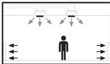
Bild 6.3: Kolbenlüftung II (Fa. FfH – Fachplanung für Haustechnik)
