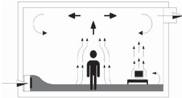
Bild 6.4: Wirkprinzip der Quelllüftung (Fa. FFH – Fachplanung für Haustechnik)
