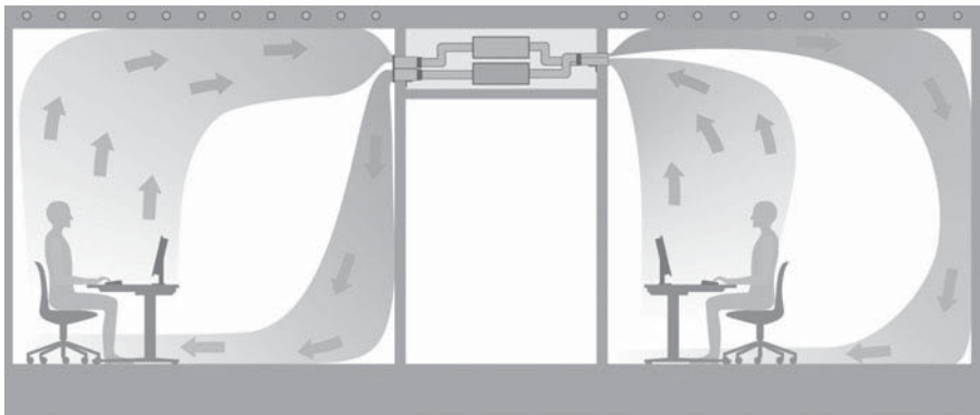
Bild 6.11: Funktionsweise des kombinierten Quellluftauslasses (Fa. TROX GmbH)
