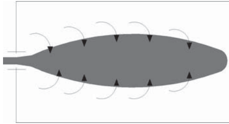
Bild 6.5: Freistrahls (Fa. FfH – Fachplanung für Haustechnik)
