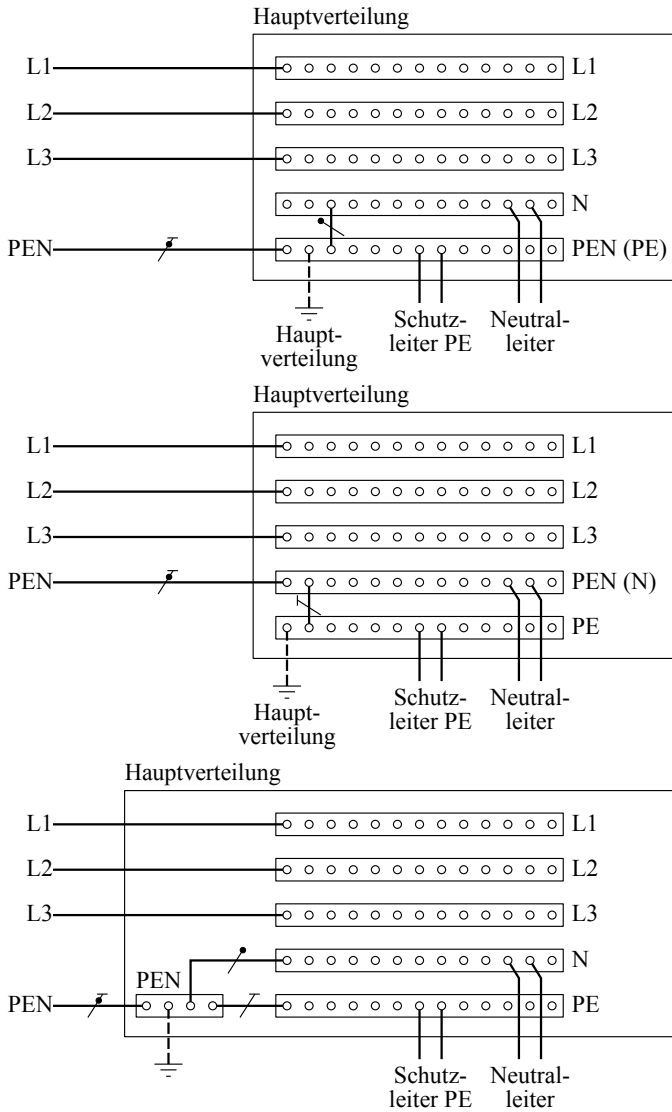
Bild 12.1 Anschluss des PEN-Leiters des einspeisenden Versorgungsstromkreises mit Aufteilung dieses Leiters in Schutzleiter und Neutralleiter in der Hauptverteilung (Quelle: DIN VDE 0100-540:2012-06, Bild 54.1)
