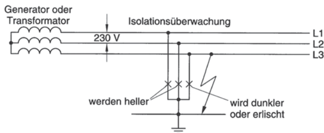
Bild 2.8 Isolationsüberwachung mit Lampen (Prinzipschaltbild)
