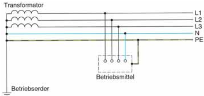
Bild 2.2 TN-S-System
