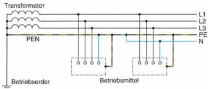
Bild 2.4 TN-C-S-System
