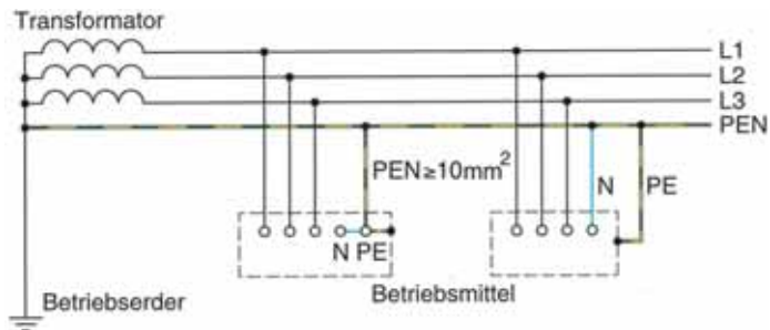
Bild 2.3 TN-C-System
