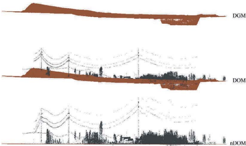
Abb. 19.1: Darstellung der Derivate DGM, DOM und nDOM aus LiDAR-Daten (Quelle: WICHT 2012)
